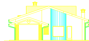
PROSPETTO LATERALE SINISTRO
