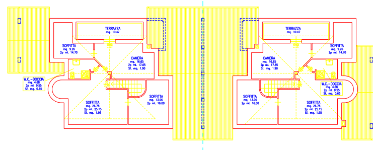
PIANTA SOTTOTETTO
